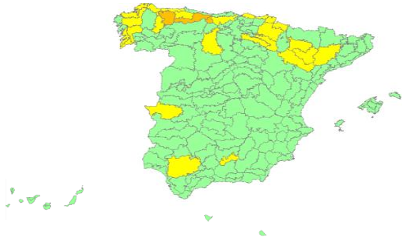
Nivel de alerta por provincias y zonas isoclimáticas Probabilidad de exceso de mortalidad atribuible a temperatura (índice Kairós)
